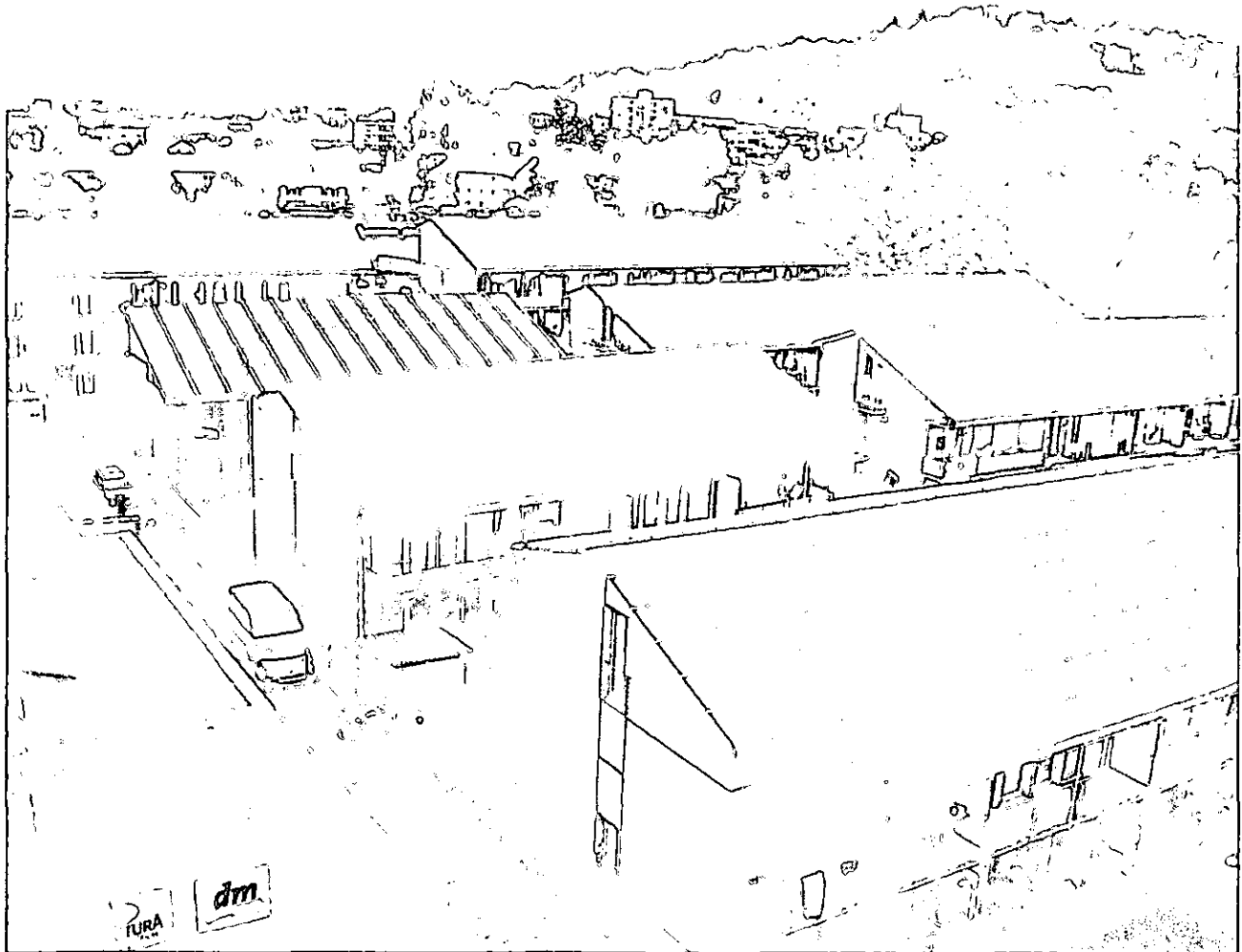
Foto 14. Vista superior de la techumbre con paneles fotovoltaicos de la Aldea Solar am Schlierberg, Freiburg
